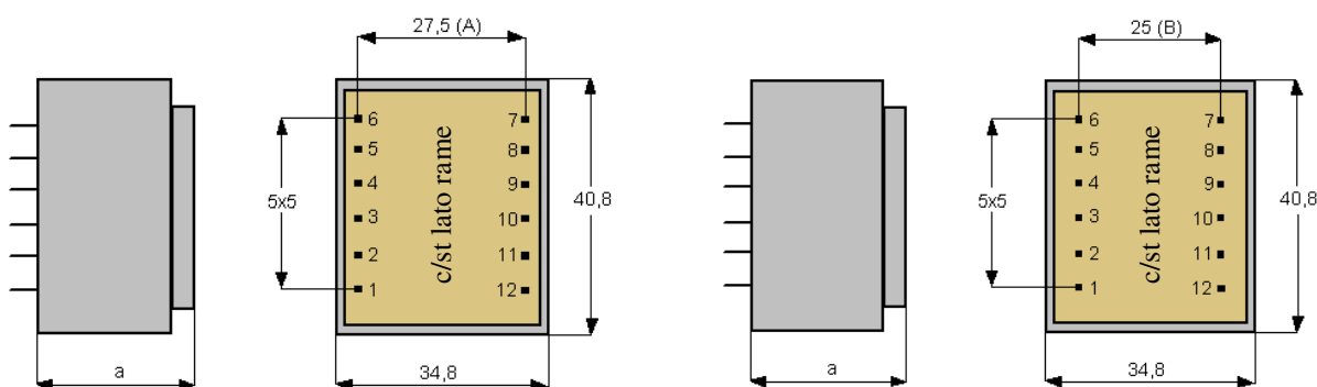
PUNTALI DI COLLEGAMENTO Ø 0,8
